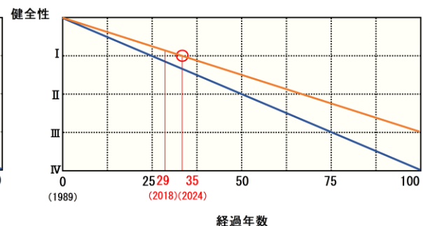
図-9 尻高カルバートの劣化予測線
