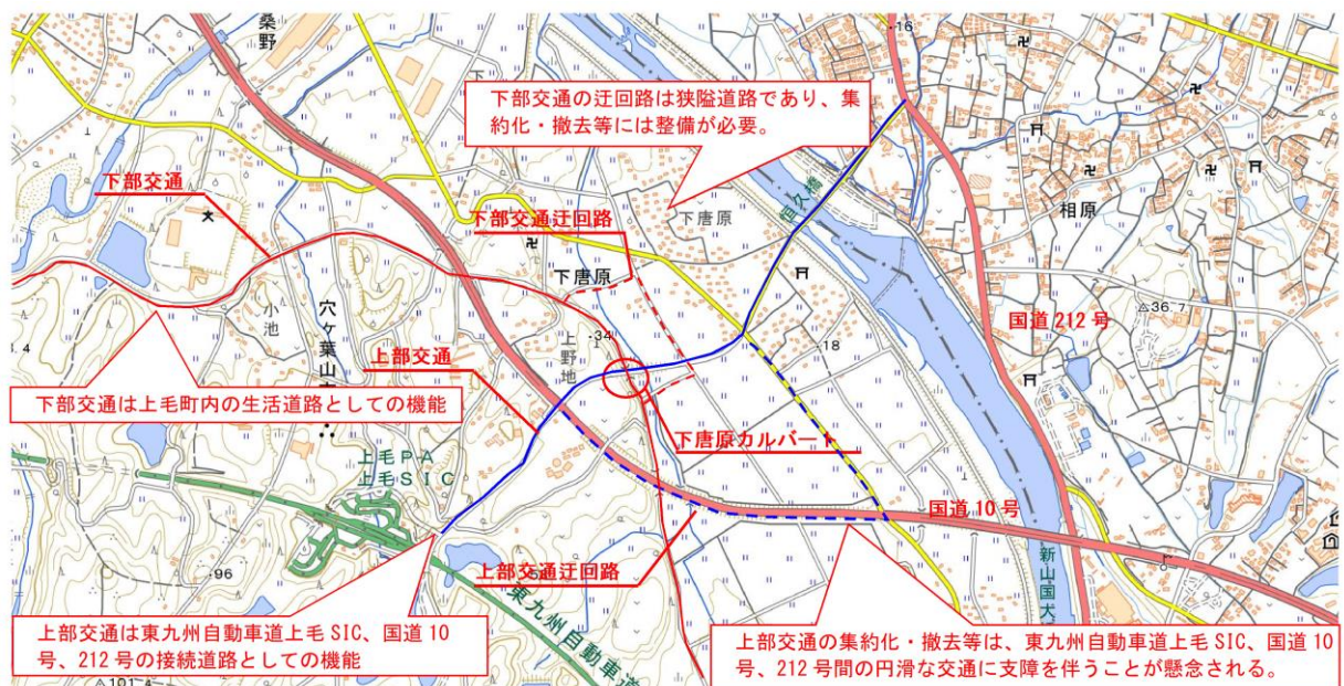
図-5 下唐原カルバートの周辺状況
