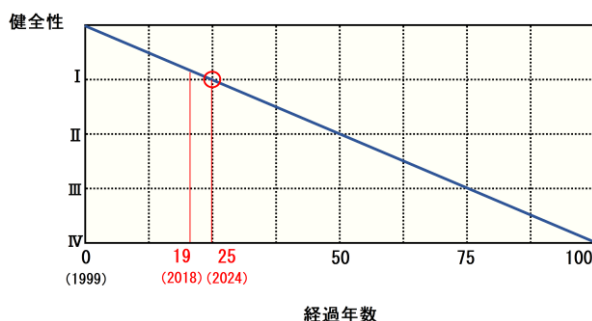
図-8 下唐原カルバートの劣化予測線
